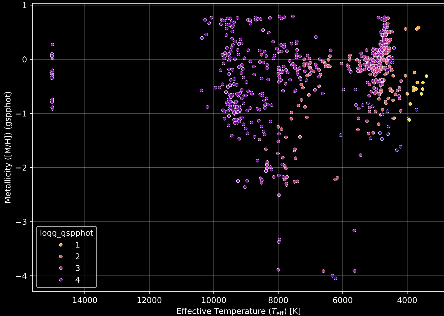
APOGEE DR17 Field: [300+00] Stellar Population Parameters (n= 682)
